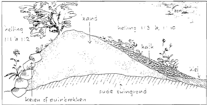
Doorsnede van een kalkhelling
